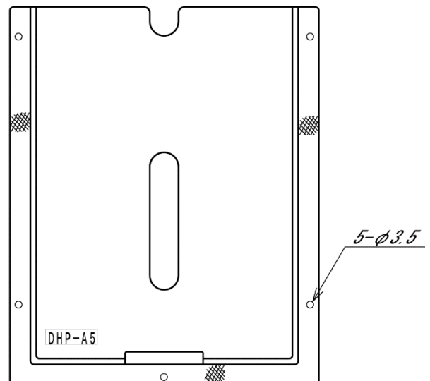
DHP-A5 変更後
