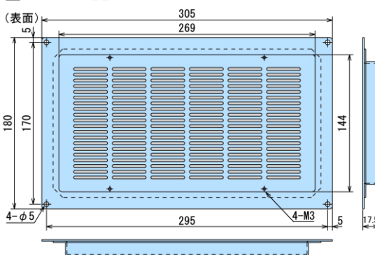
■VTU-122
