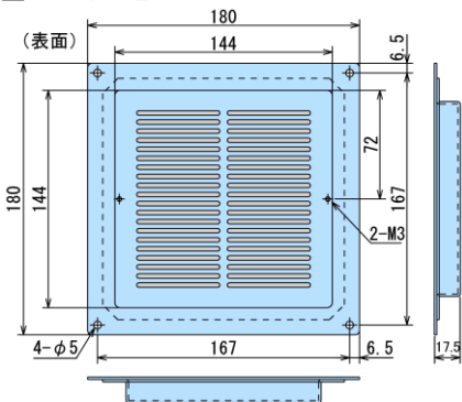
■VTU-121
