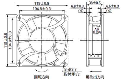
■ファン仕様
