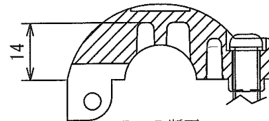
B-B断面
