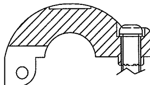
A-A断面
