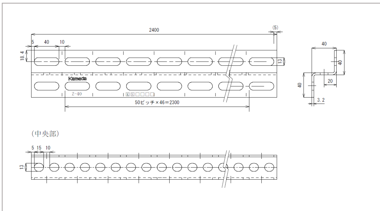
図面B (旧型) Z-40
