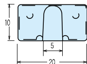
■ ED-20GN (3C) ■ ED-20M-3C
