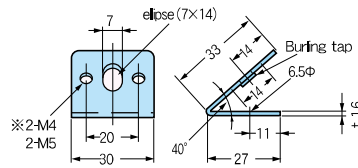
■S-1-4-3C※ (M4) ■S-1-3C (M5)
