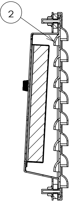
断面図 A-A スケール 1 : 3
