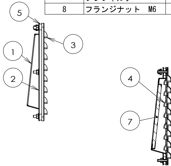
断面図 A-A
