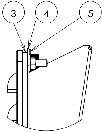
詳細図 A スケール 1 : 2
