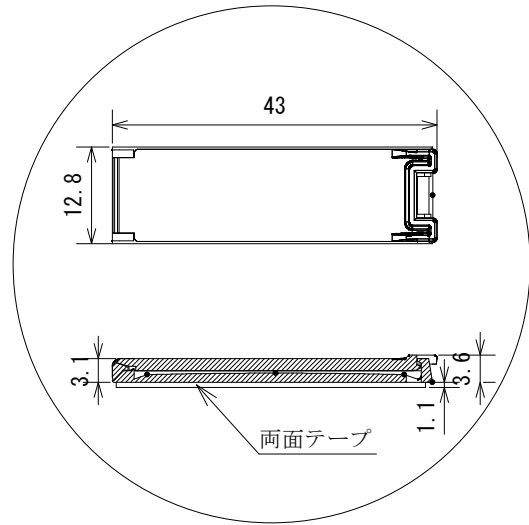
組立図
