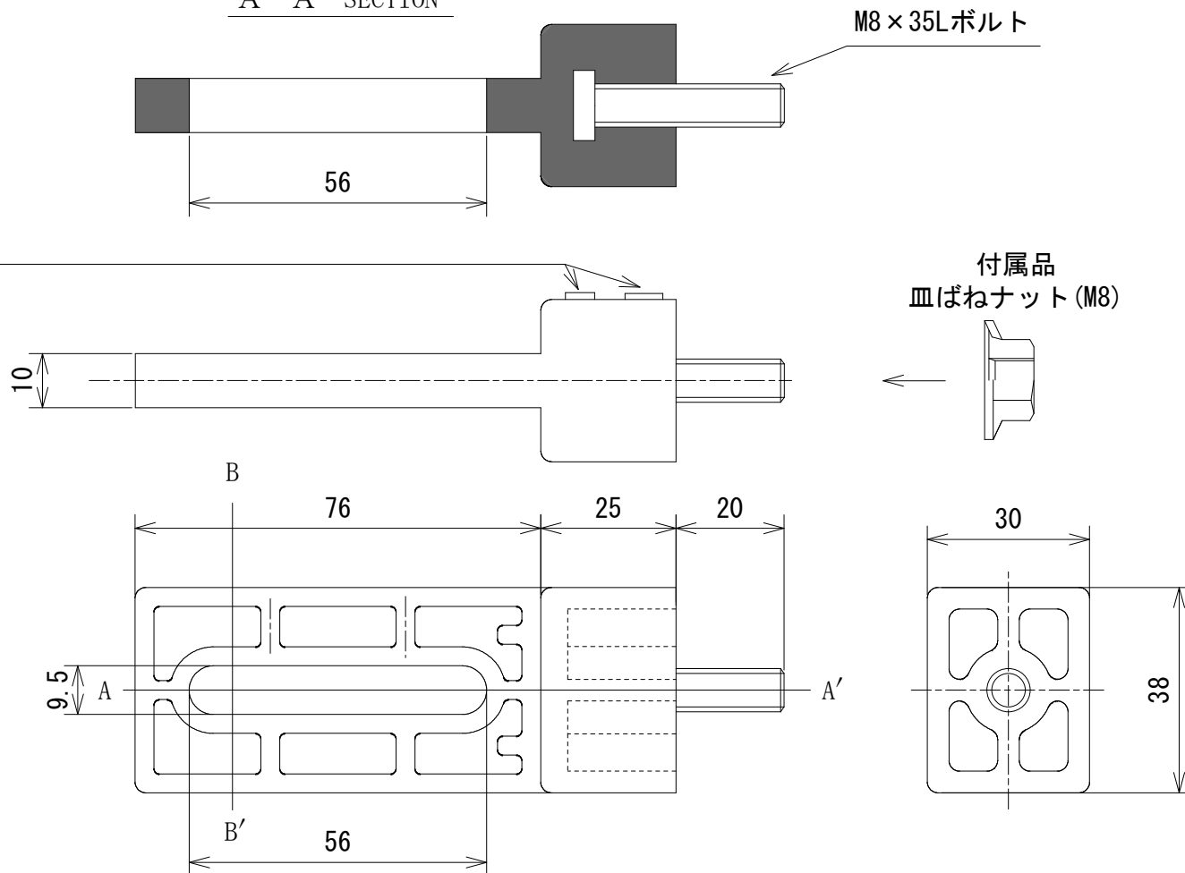
A - A' SECTION
